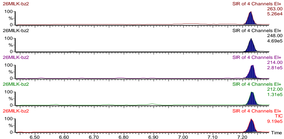
图 A1 氯羟吡啶标准溶液离子色谱图 (20 ng/mL)
