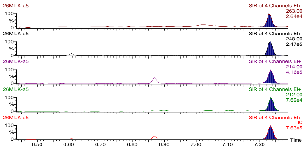
图 A3 牛奶空白添加氯羟吡啶试样离子色谱图 (10 µg/kg)
